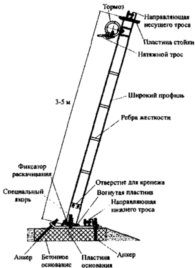
Рис. 34. Стойка барьера
