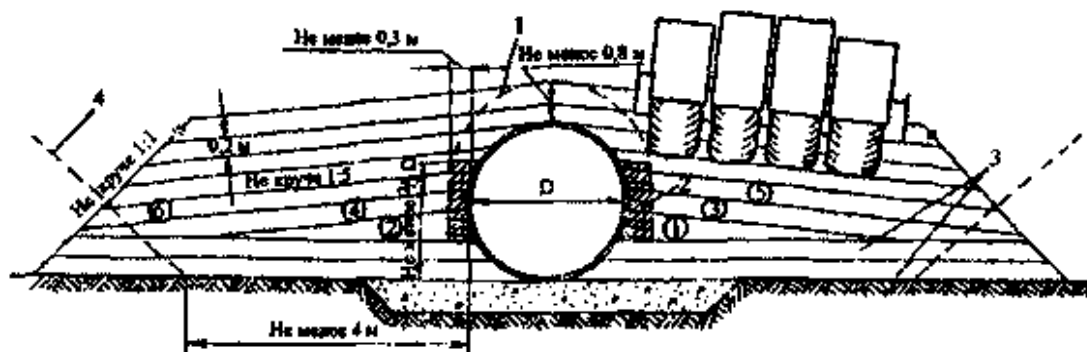
Рис. 26. Технологическая последовательность и схема послойного уплотнения грунта засыпки МГТпневмокатками:
