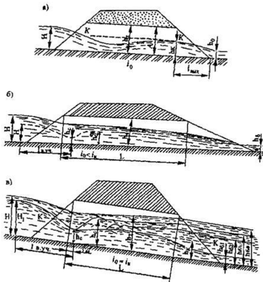
Рис. Е.3. Схема протекания воды в равнинной МГТ при безнапорном режиме:
