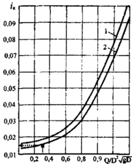
Рис. 5.27. График для определения критического уклона i_k для круглых гофрированных труб с гладкими лотками ( n_{св} = 0,025 ):
