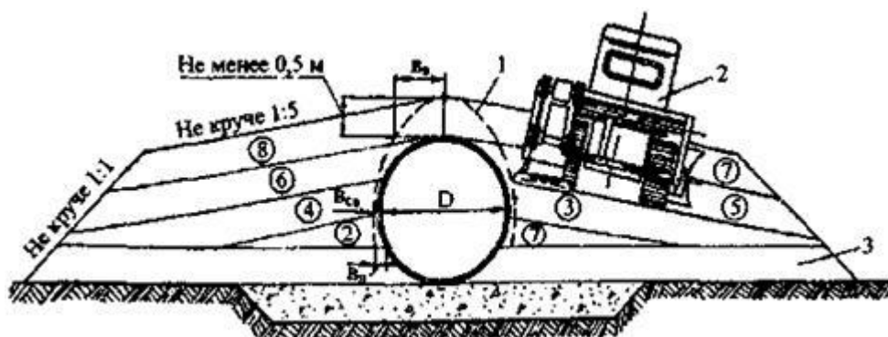
Рис. 25. Технологическая последовательность и схема послойного уплотнения грунта засыпки МГТвиброударной машиной для стесненных условий:
