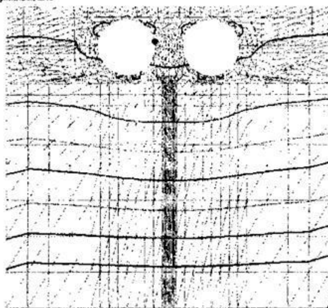
Рис. И.6. Вертикальные напряжения, кПа
