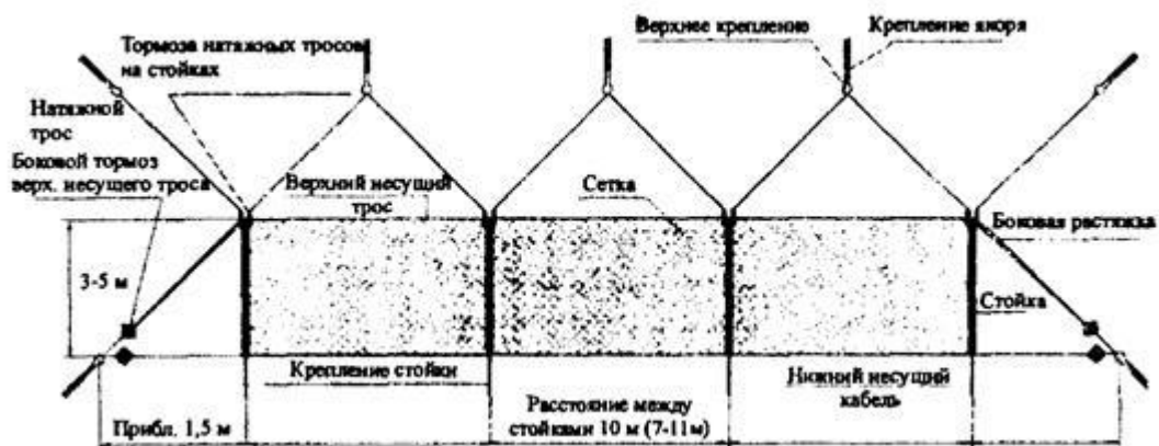
Рис. 35. Конструкции противоселевых, противокарчевых и противоледоходных барьеров
