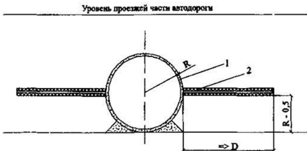
Рис. 9. Конструкция горизонтальных упоров из объемной георешетки:
