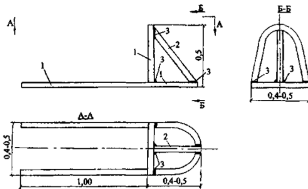
Рис. 29. Конструкция выдвижного стабилизатора:
