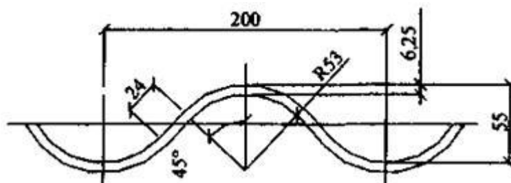
Рис. А.5. Профиль гофрированного листа
