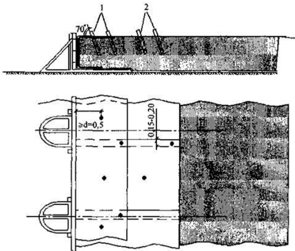
Рис. 32. Укладывание с натяжением на уплотненную поверхность грунта выпущенных за внешнюю грань щитов армирующих полотнищ и закрепление их кольщиками:
