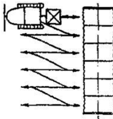
Рис. 24. Схема уплотнения грунта виброударной машиной челночным способом
