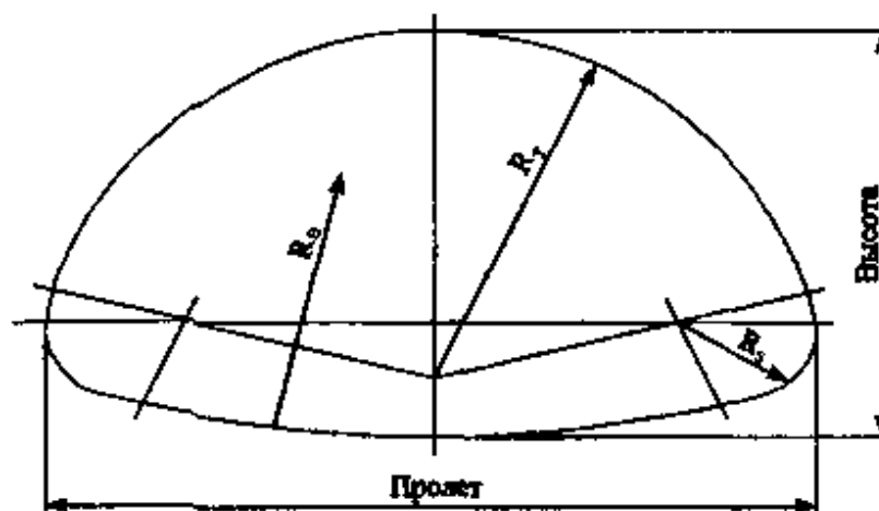
Рис. 4. МГТ замкнутого арочного типа
