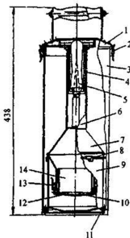
Рис. Л.1. Схема плотномера-влажномера Н.П. Ковалева:
