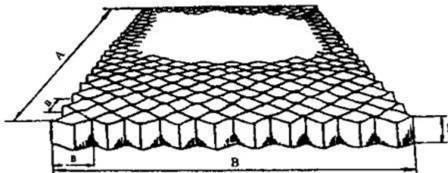
Рис. 15. Общий вид георешетки в рабочем (растянутом) состоянии
