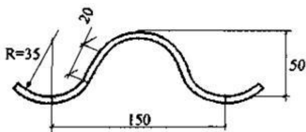
Рис. А.3. Профиль гофрированного листа
