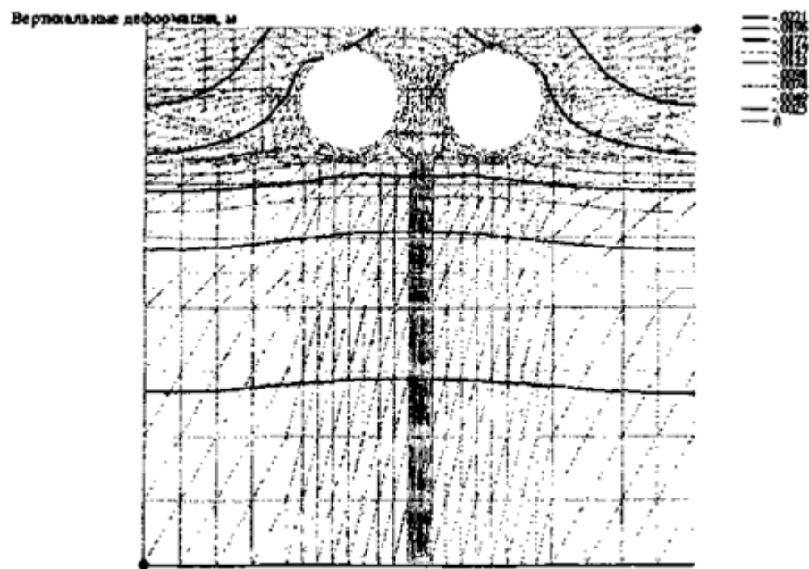
Рис. И.4. Вертикальные деформации, м
