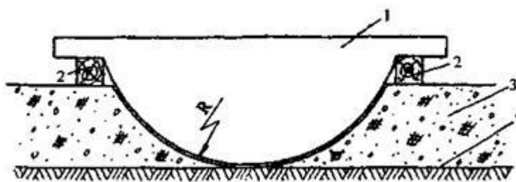
Рис. 14. Вырезка грунтового ложа по шаблону:
