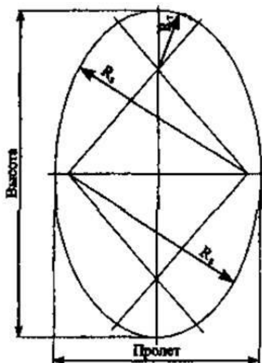
Рис. 3. МГТ формы вертикального эллипса
