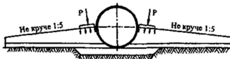
Рис. 22. Схема засыпки и уплотнения грунта наклонными слоями
