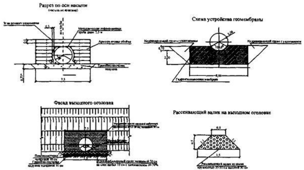
Рис. М.2. Пример проектирования армогрунтовой обшивки, противофильтрационного экрана(геомембраны), входного и выходного оголовка и рассеивающего валика для МГТ на рис. М.1
