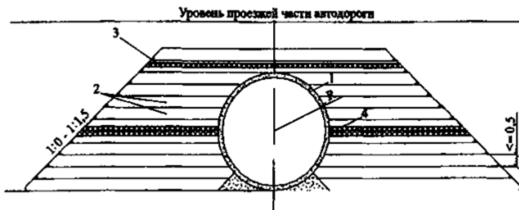
Рис. 10. Конструкция обоймы из армированного грунта:
