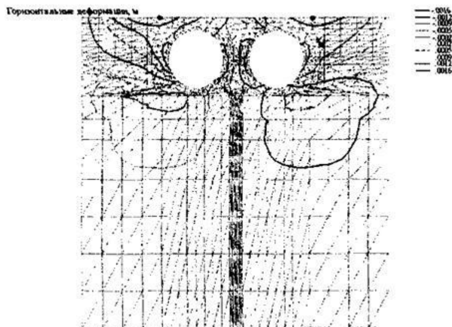
Рис. И.5. Горизонтальные деформации, м
