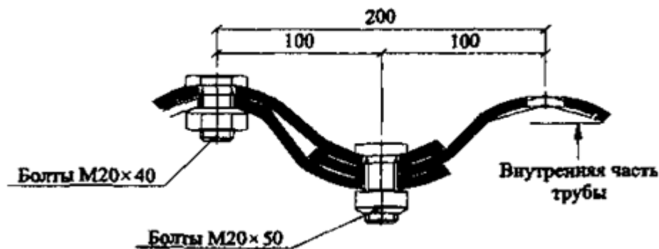
Рис. Б.3. Перекрытие листов
