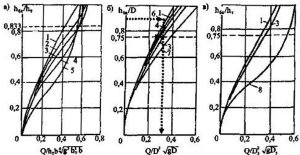
Рис. 5.19. Графики для определения глубины воды на входе в прямоугольные (а), круглые (б) и овоидальные (в) трубы при типах оголовков:
