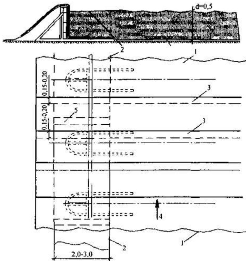
Рис. 31. Установка стабилизаторов, закрепление щитов, расстилка армирующих полотнищ и геотекстиля отсыпка слоя армогрунта:
