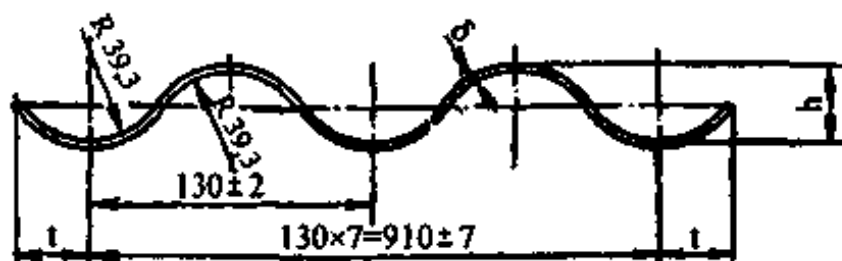
Рис. А.1. Профиль гофрированного листа
