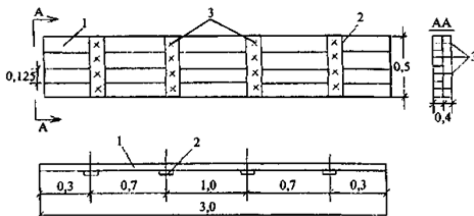
Рис. 30. Конструкция лицевого щита:
