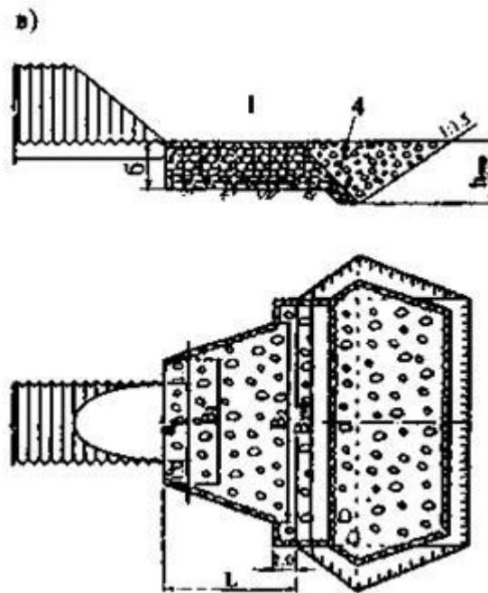
Рис. Е.4. Типы выходных русл из каменной наброски:
