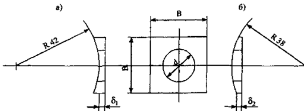
Рис. Б.1. Шайбы для болтов (размеры в миллиметрах):
