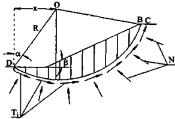
Рис. Ж.2. Принципиальная схема метода КЦПС
