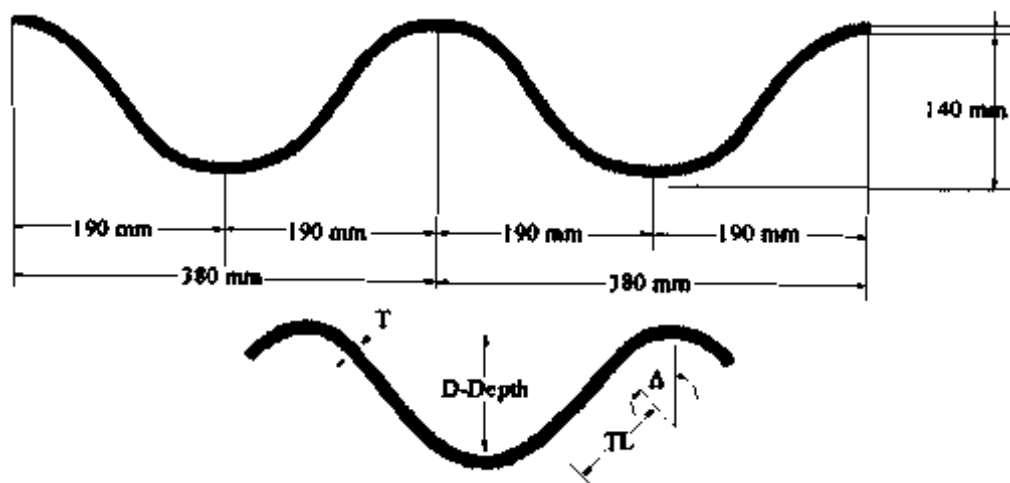
Рис. А.4. Профиль гофрированного листа
