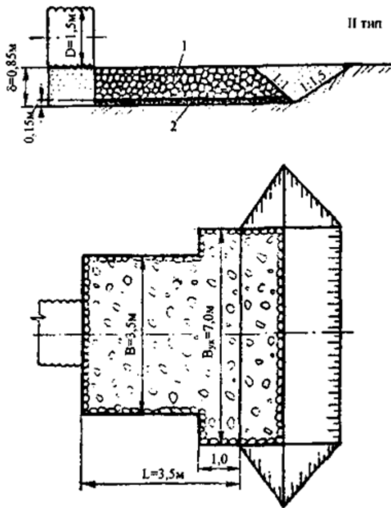
Рис. Е.5. Конструкция укрепления:
