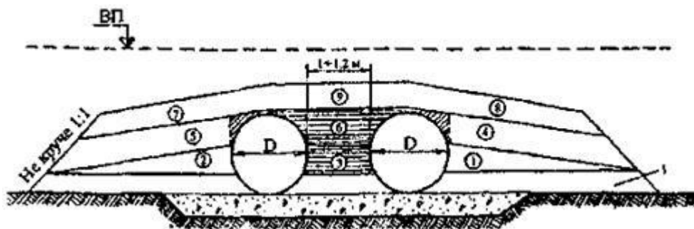
Рис. 27. Технологическая последовательность и схема послойного уплотнения грунта засыпочно-гооочковых МГТ:
