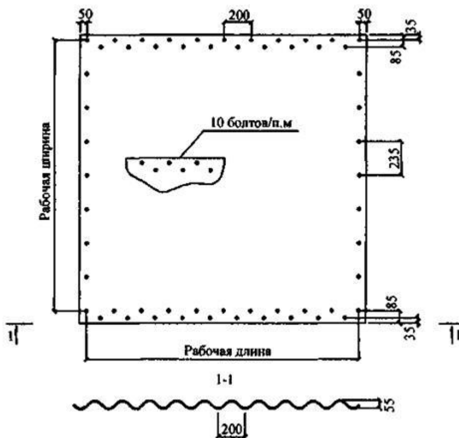
Рис. А.5. Профиль гофрированного листа
