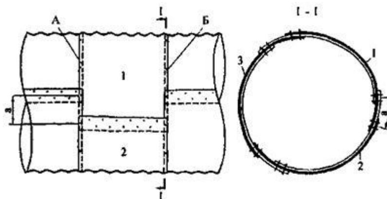
Рис. 18. Схема соединения двух секций соединительными элементами:
