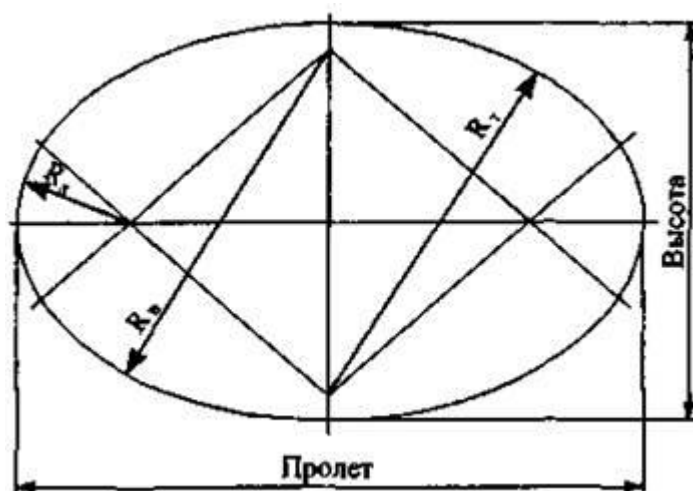
Рис. 2. МГТ формы горизонтального эллипса
