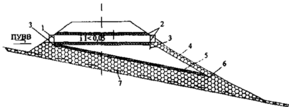
Рис. 12. Устройство МГТ на косогоре:
