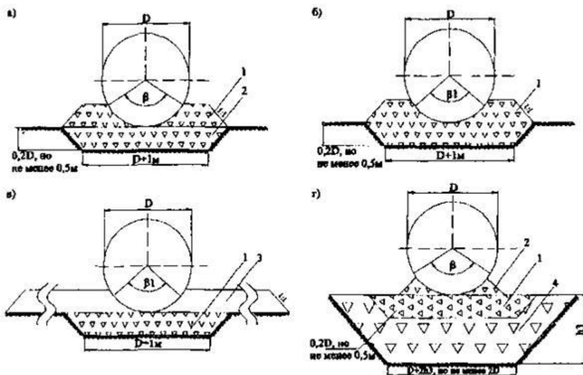
Рис. 7. Конструкция основания:
