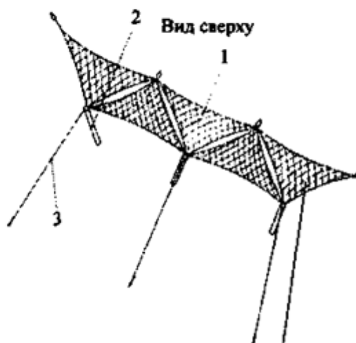
Рис. 37. Конструкции противоналедных сеток:
