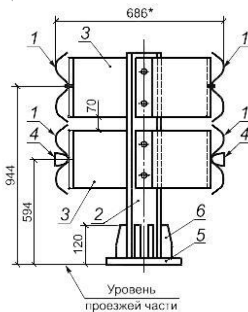
д) Двухстороннее двухъярусное ограждение
