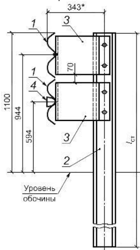
в) Одностороннее двухъярусное ограждение
