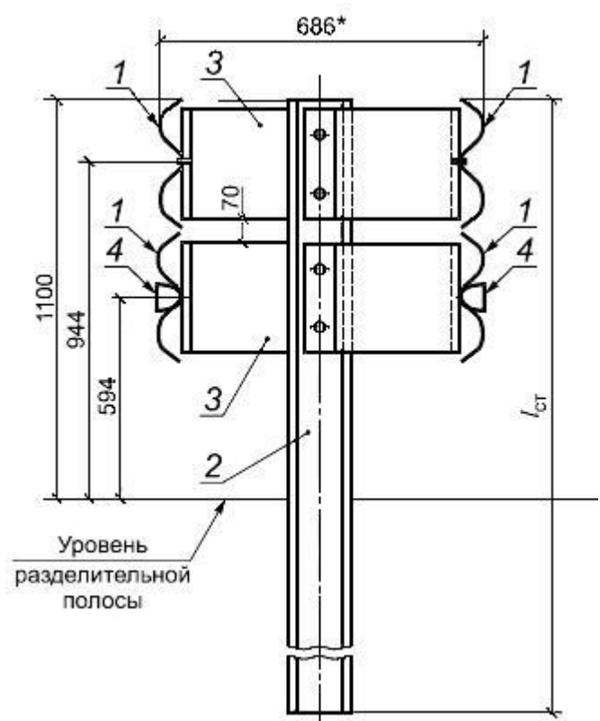
г) Двухстороннее двухъярусное ограждение
