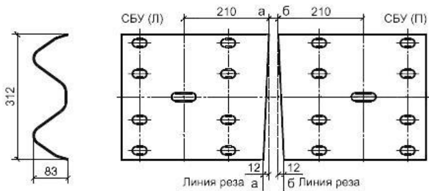
Рисунок 5 - Секция балки угловой СБУ
