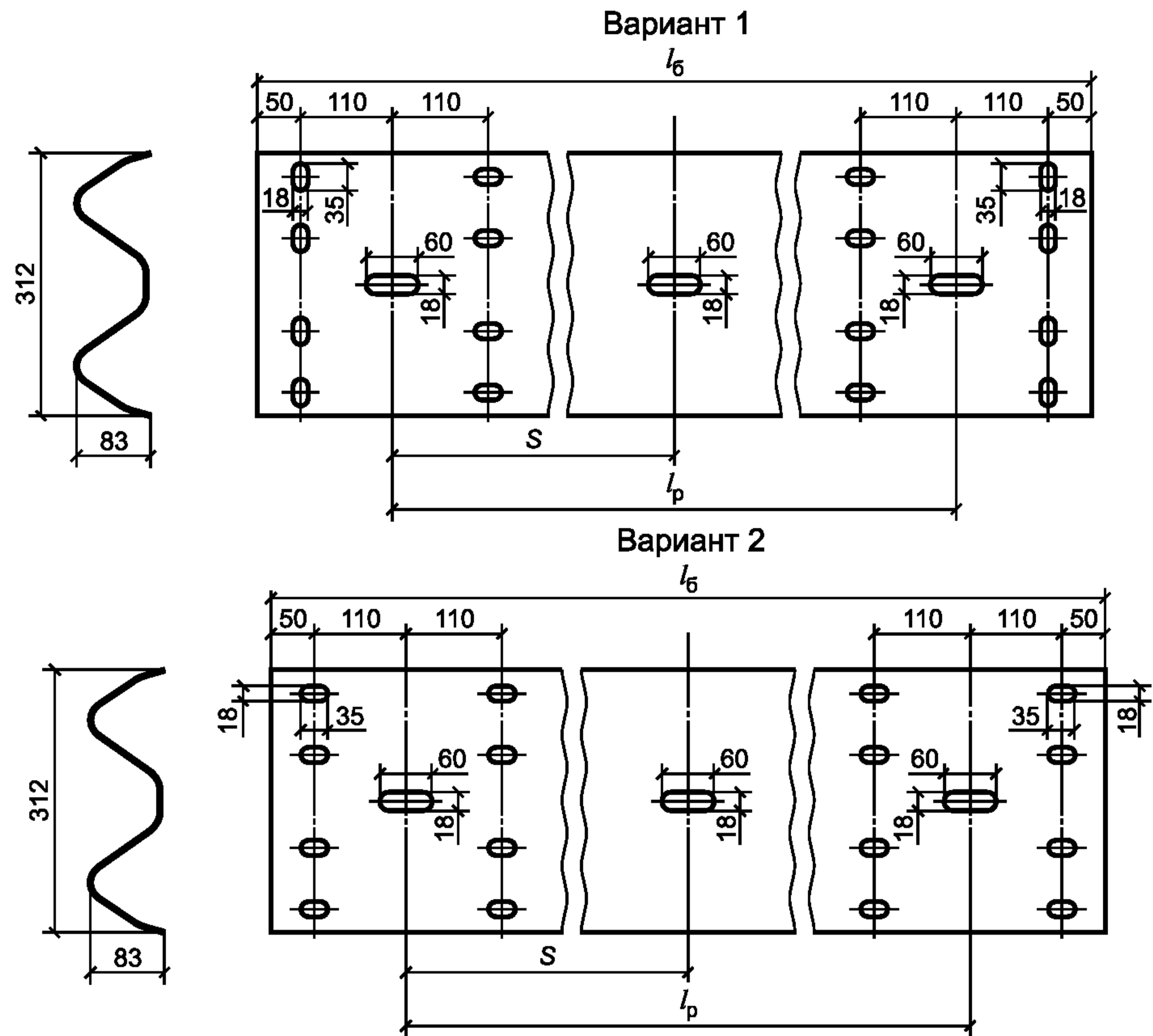
Рисунок 4 — Секция балки ограждений СБ
