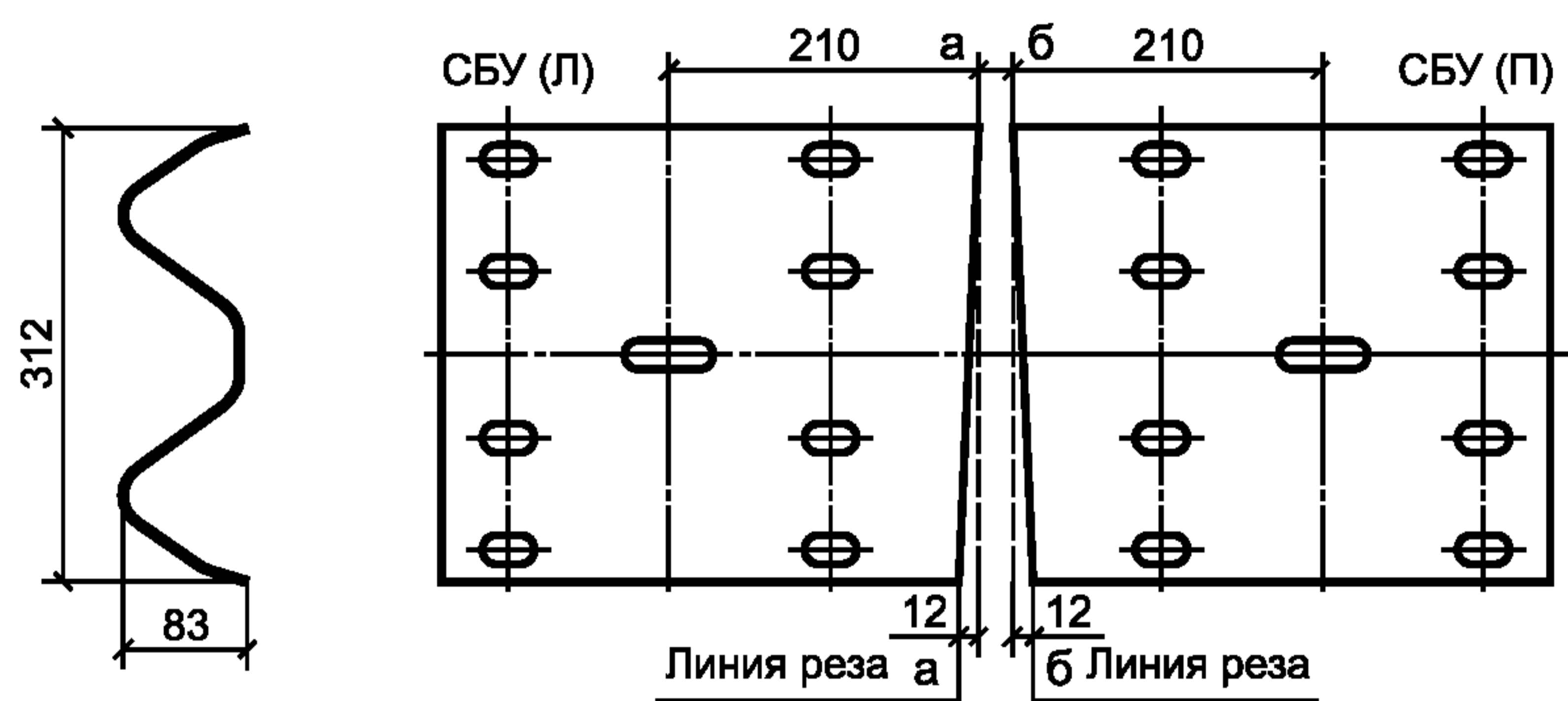
Рисунок 4 — Секция балки ограждений СБ
