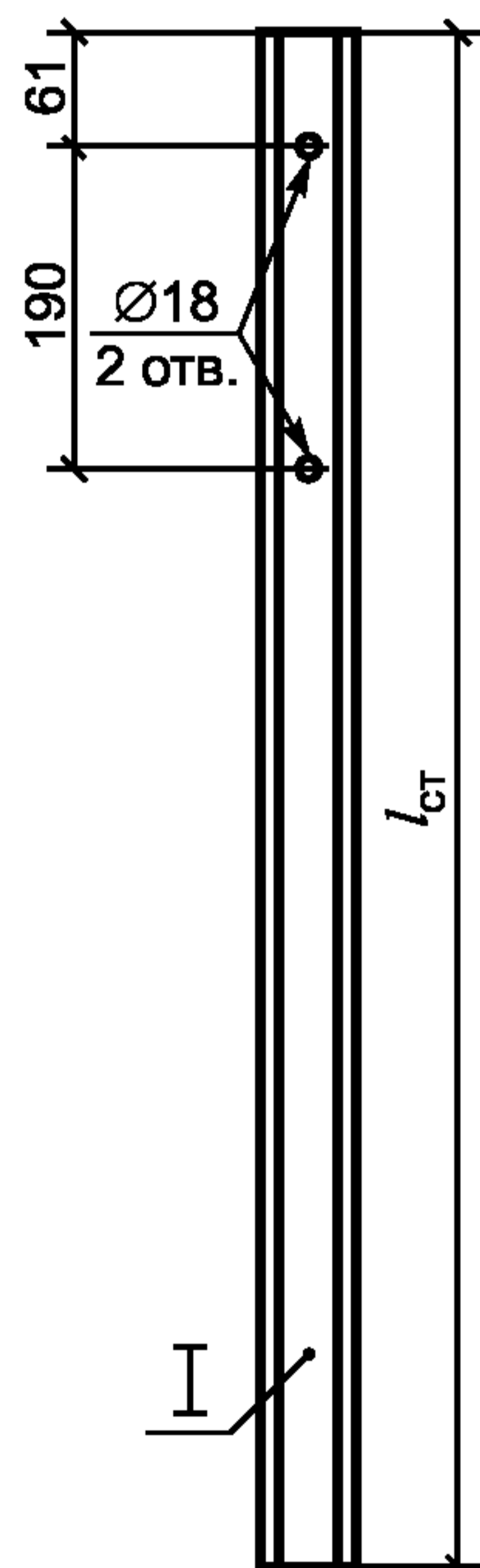
а) Для односторонних ограждений с жесткими консолями
