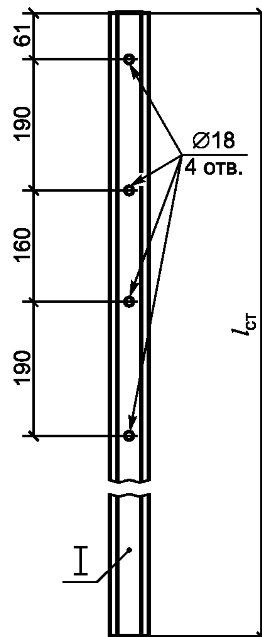
в) Для двухсторонних ограждений с консолью-распоркой
