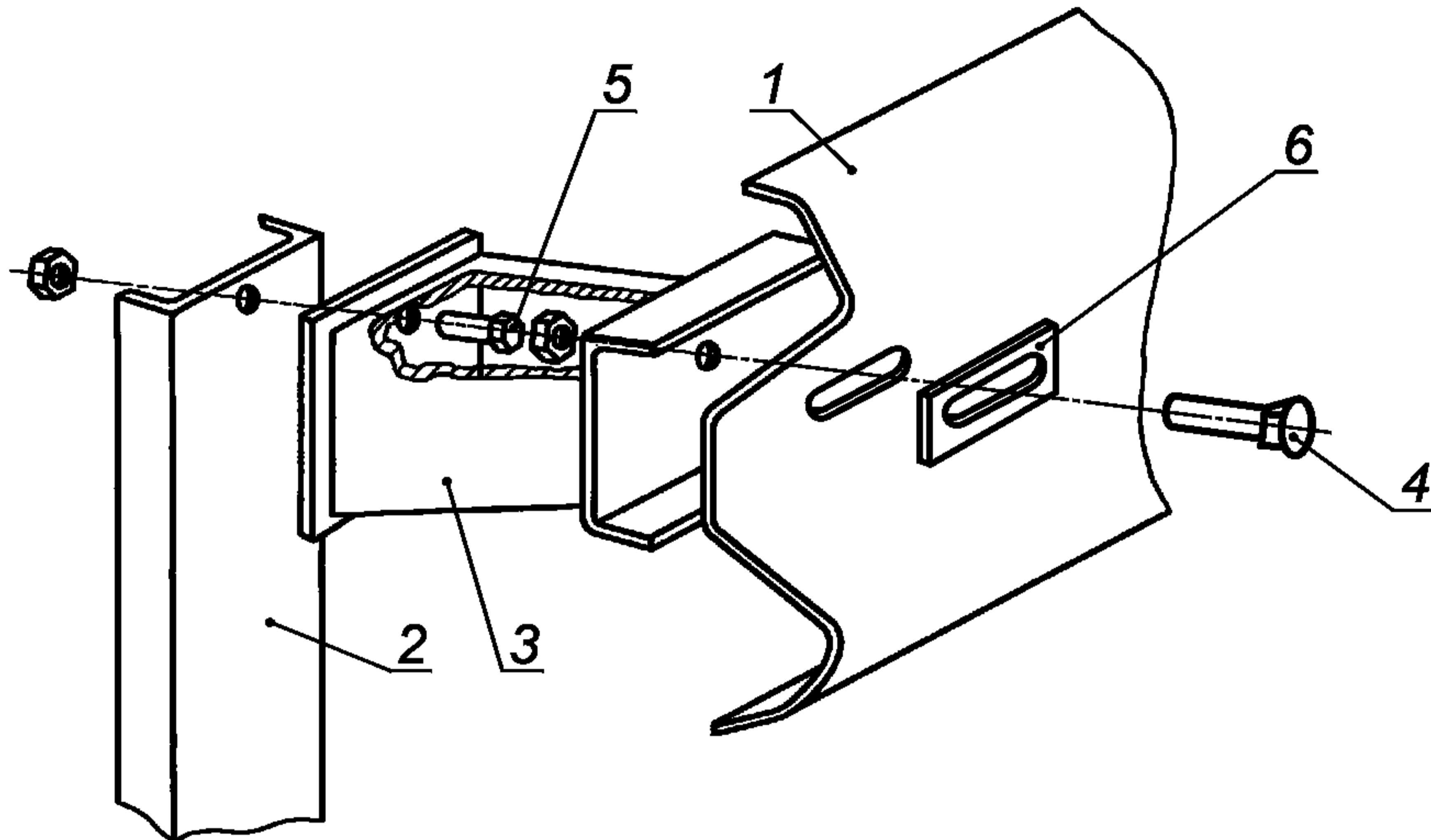
1 — балка; 2 — стойка; 3 — консоль жесткая, 4 — болт M16 × 45.5.8; 5 — болт M16 × 30.5.8; 6 — шайба 80 × 40 × 4 мм
