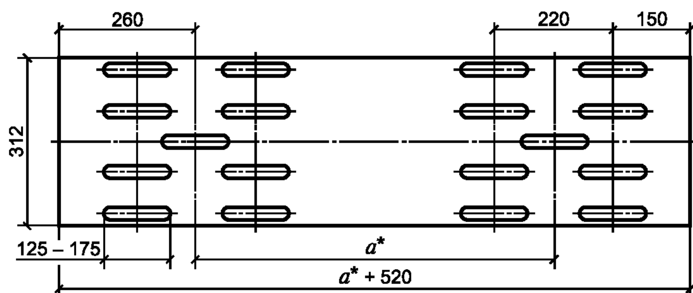
Рисунок 5 — Секция балки угловой СБУ
