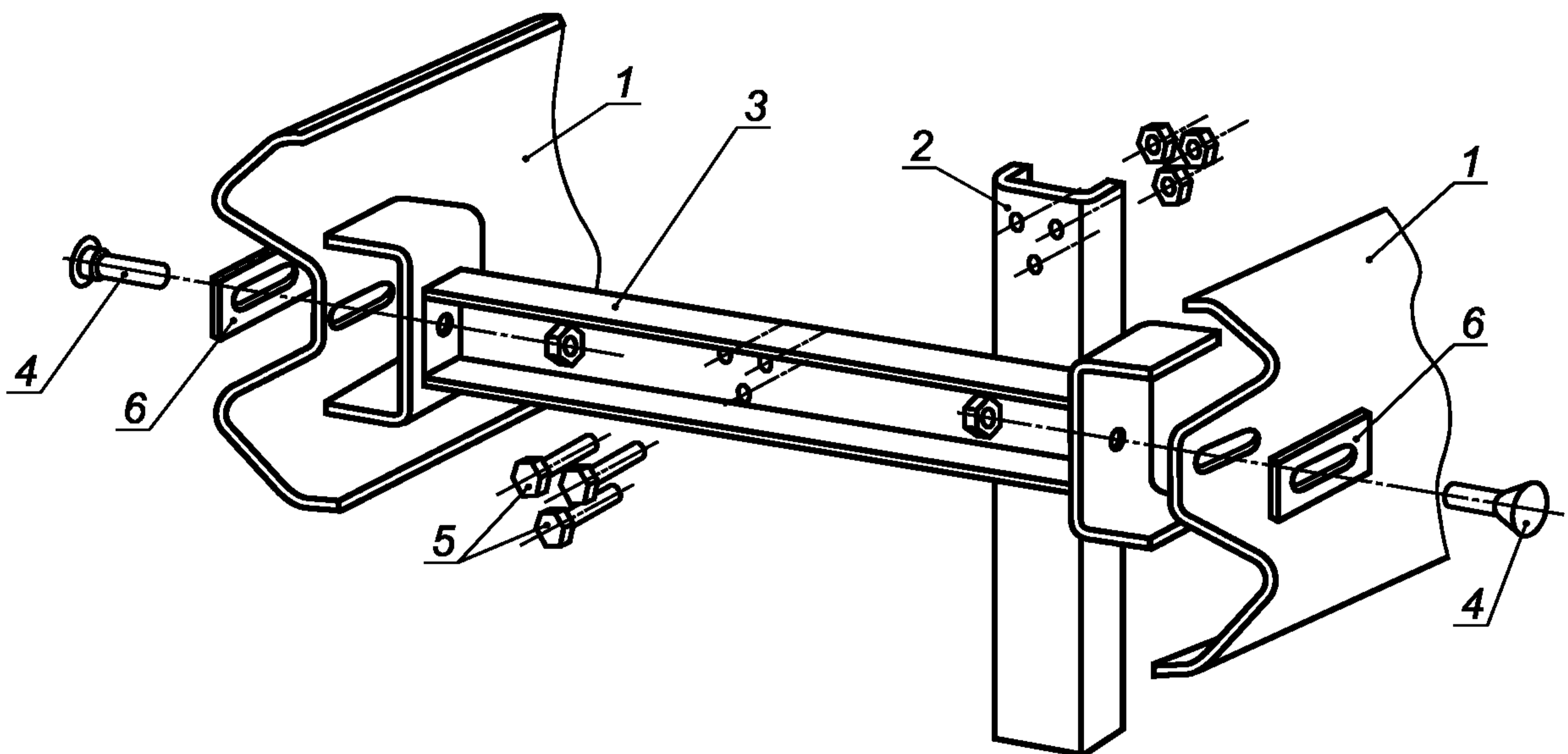
1 — балка; 2 — стойка; 3 — консоль-распорка; 4 — болт M16 × 45.5.8; 5 — болт M16 × 30.5.8; 6 — шайба 80 × 40 × 4 мм
